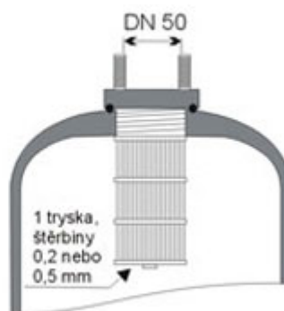
Horní systém - PP příruba DN 50
