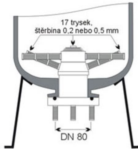
Spodní systém - PP příruba DN 80
