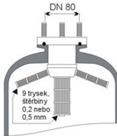
Horní systém - PP příruba DN 80
