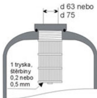
Horní systém - objímka PVC d 63 nebo d 75 kolmo k nalepení
