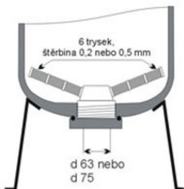
Spodní systém - objímka PVC d 63 nebo d 75 kolmo k nalepení
