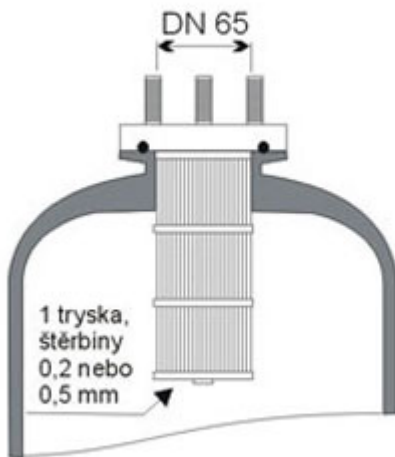
Horní systém - PP příruba DN 65
