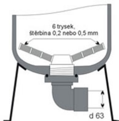
Spodní systém - koleno d 63 k nalepení
