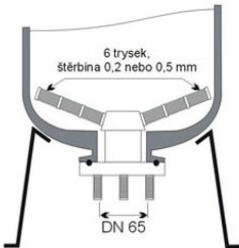
Spodní systém - PP příruba DN 65
