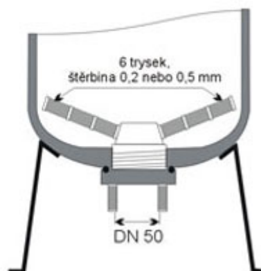
Spodní systém - PP příruba DN 50
