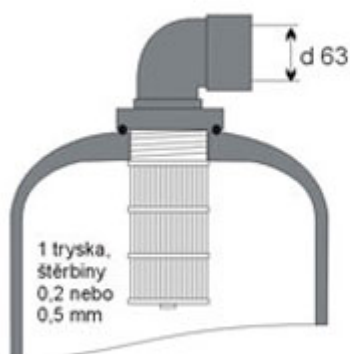
Horní systém - koleno d 63 k nalepení
